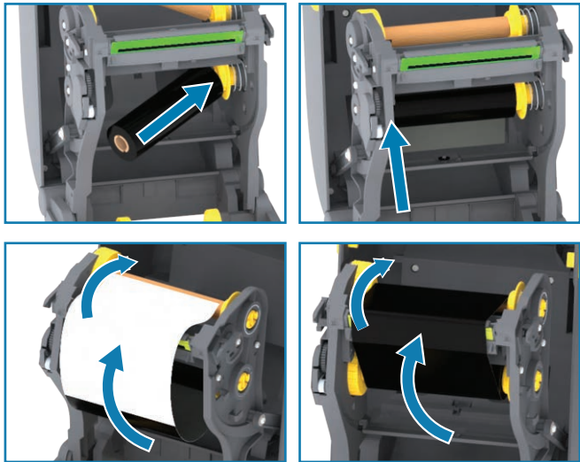
将色带装入底部转轴 拉动色带引头并将其接到拾取芯上。向前卷动。
